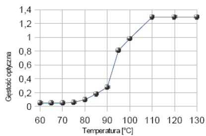
Czułość statyczna
