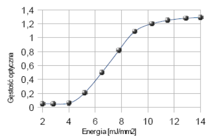
Czułość dynamiczna
